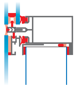
Bild 22. Limmad infästning (structural glazing).
