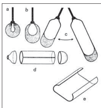
Bild 5. Framställning av glas enligt cylindermethoden.
