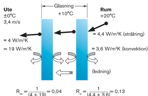
Bild 47. Förutsättningar för beräkning av värmeöverföring via strålning, konvektion och ledning. R_{se} = yttre värmeöverföringstal, R_{si} = inre värmeöverföringstal.
