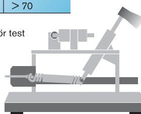
Bild 38. Yxtest.
