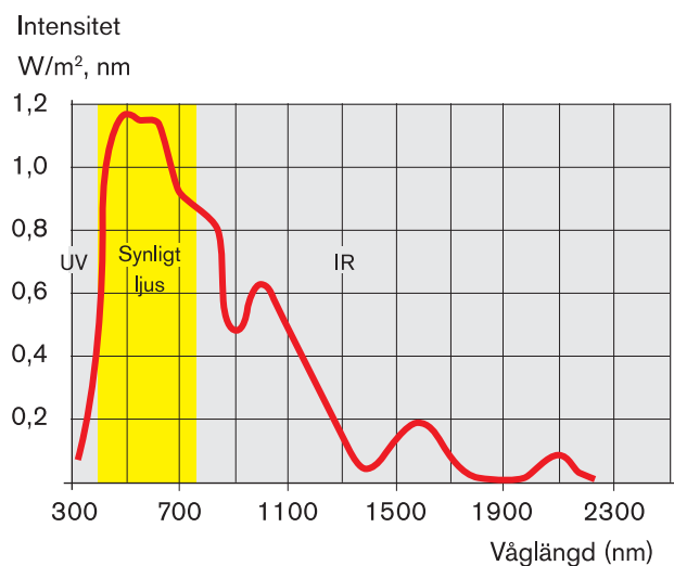
Bild 11. Solstrålningens fördelning.
