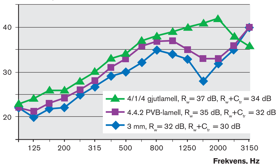
Reduktionstal, dB
